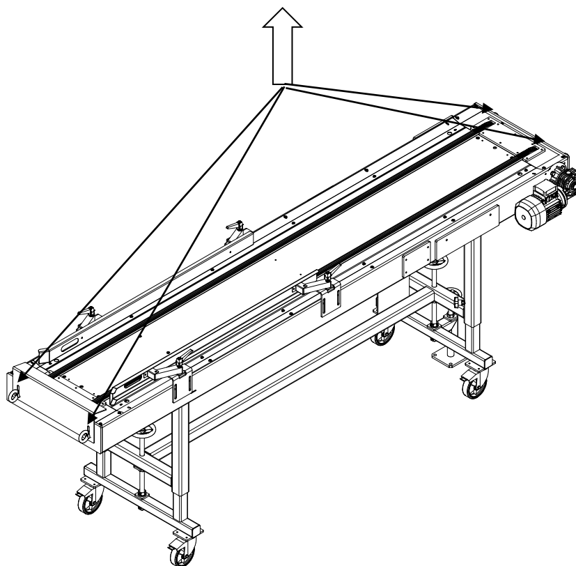
Punti di sollevamento Lifting points
