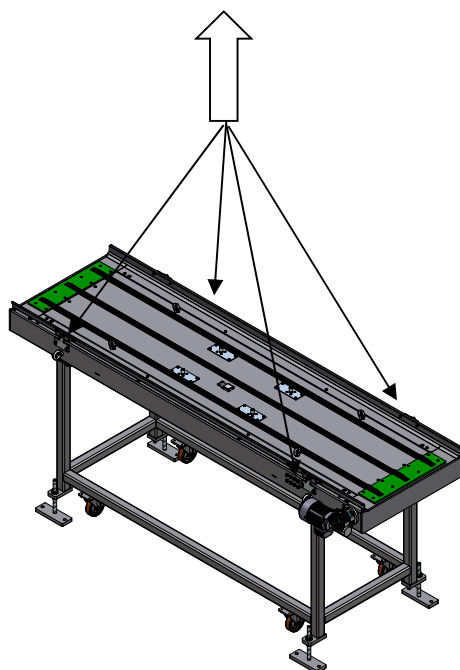
Punti di sollevamento Lifting points
