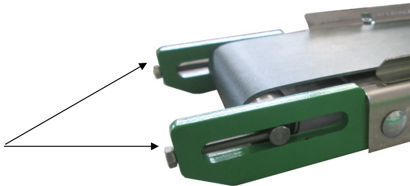
Vite regolazione rullo Roller adjustment screw
